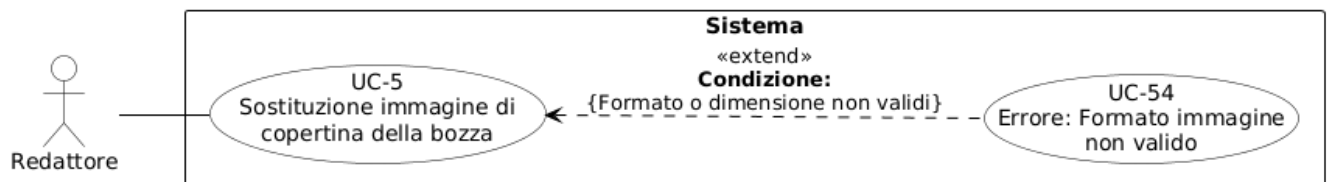
Figura 12: Diagramma del caso d'uso UC-5: Sostituzione immagine di copertina della bozza
