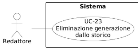
Figura 30: Diagramma del caso d'uso UC-23: Eliminazione generazione dallo storico
