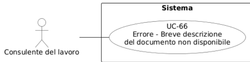
Figura 103: Diagramma del caso d'uso UC-66: Errore per breve descrizione del documento non disponibile
