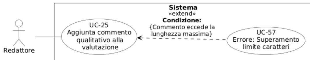
Figura 32: Diagramma del caso d'uso UC-25: Aggiunta commento qualitativo alla valutazione
